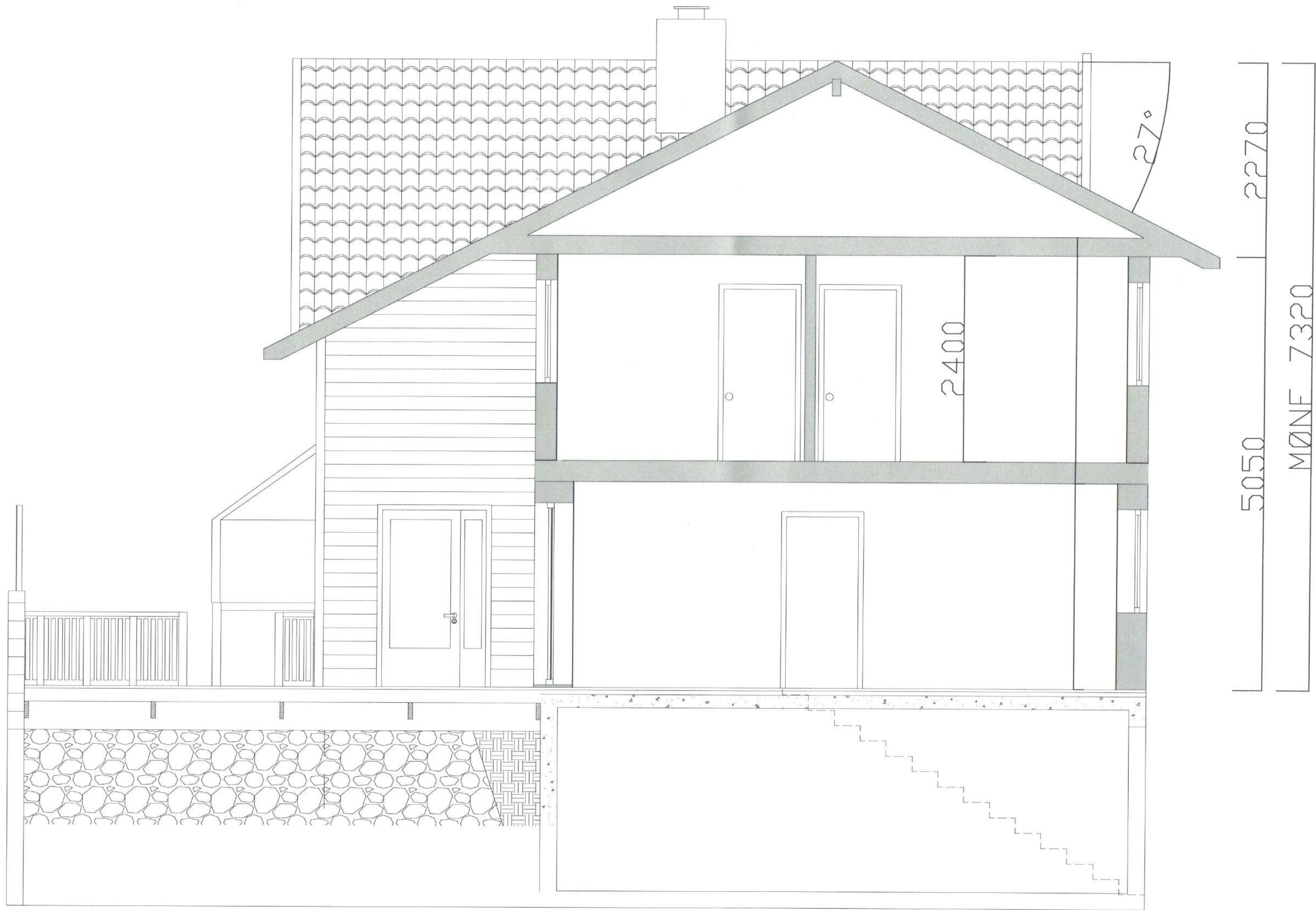
SNITT A-A
